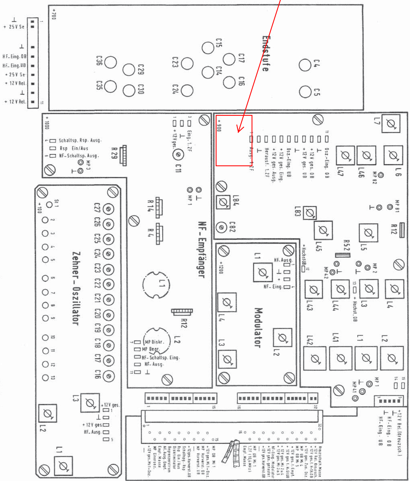
Übersicht zur Lage der Abgleich- und Meßpunkte Frontplatte (auf dem Kopf stehend) dem Betrachter zugekehrt, NF-Platte herausgeschwenkt (Sender- und Empfängerseite)
